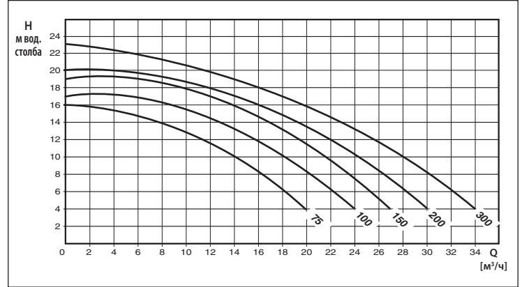
КРИВЫЕ ЭКСПЛУАТАЦИОННЫХ ХАРАКТЕРИСТИК SWT
