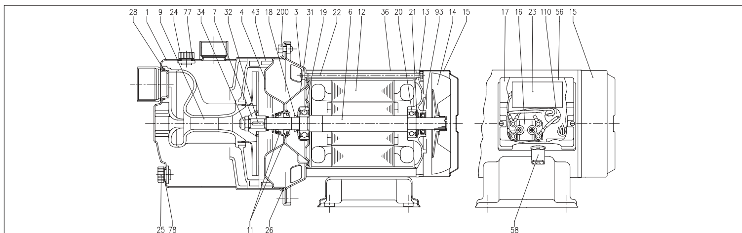
РАЗРЕЗ JE
